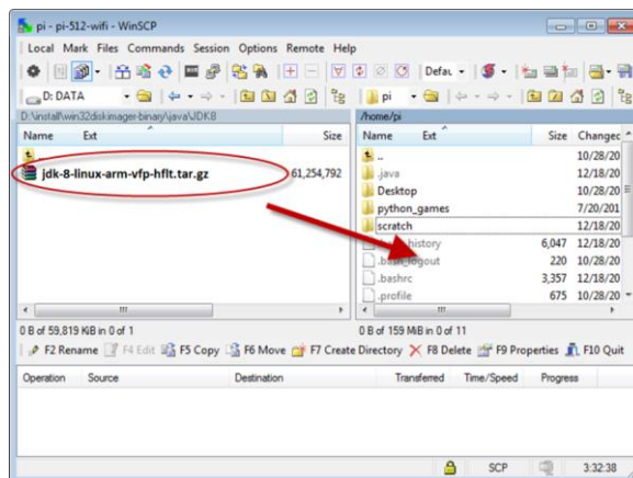
Рис.5.33 Копіювання файла Oracle JDK на Raspberry Pi
