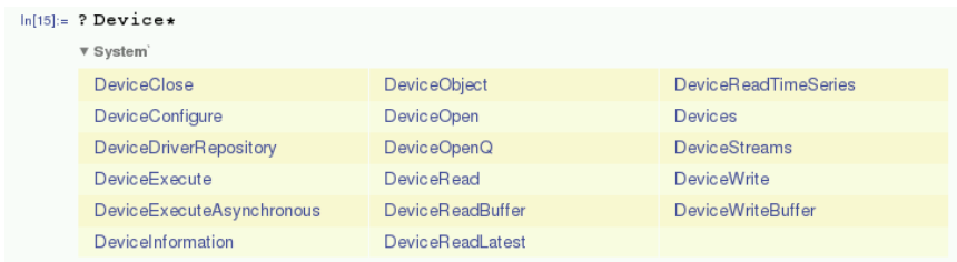
Рис.8.9 Функція пошуку
