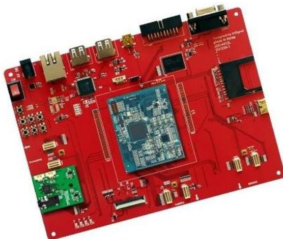
Рис.10.36 Плата Origen 4
