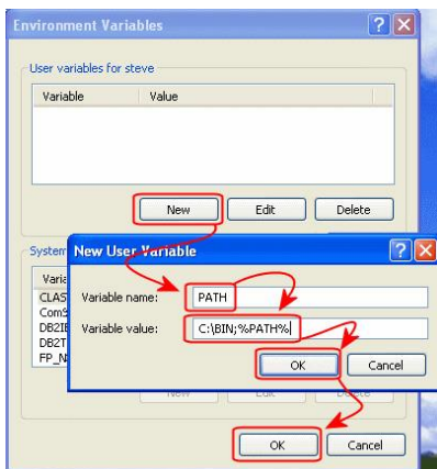
Рис.3.2 Змінні середовища
