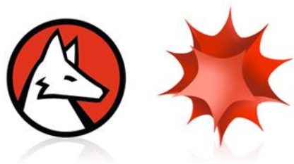
Рис.8.2 Wolfram & Mathematica
