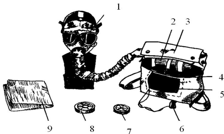
Рис. 1.197 – Ізолюючий дихальний апарат ИП-4М: 1) маска МИА-1; 2) регенеративний патрон РП-4; 3) торба; 4) каркас; 5) дихальний мішок; 6) пробка; 7) мембрани переговорного пристрою; 8) незапінтілі плівки; 9) мішок для зберігання
