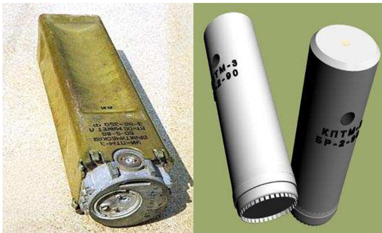
Рис. 1.178 – Протитанкова протиднищева міна дистанційного мінування ПТМ-3 та касета КПТМ-3
