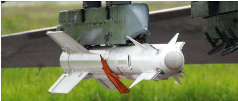
Рис. 2.83 – Ракета малої дальності Р-73
